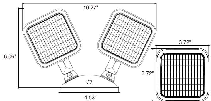
VE-RH-2(WH)
